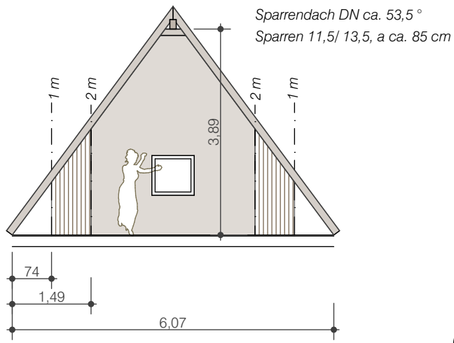
Schnitt_Dachboden 1:100
